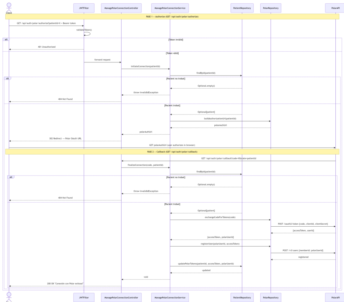
7.3.24. Diagrama de Seqüència ManagePolarConnection. Font: Elaboració pròpia
