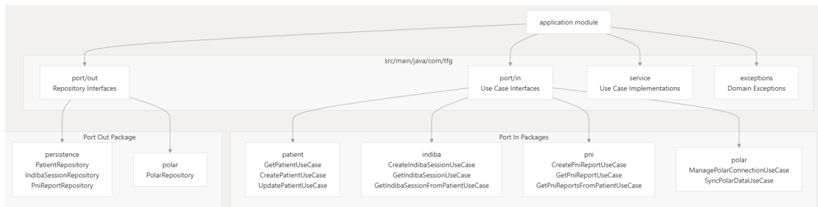
7.1.15. Diagrama de mòdul application. Font: Elaboració pròpia
