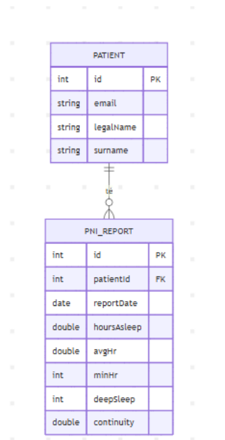
7.2.19. Diagrama d'entitat PniReport. Font: Elaboració pròpia
