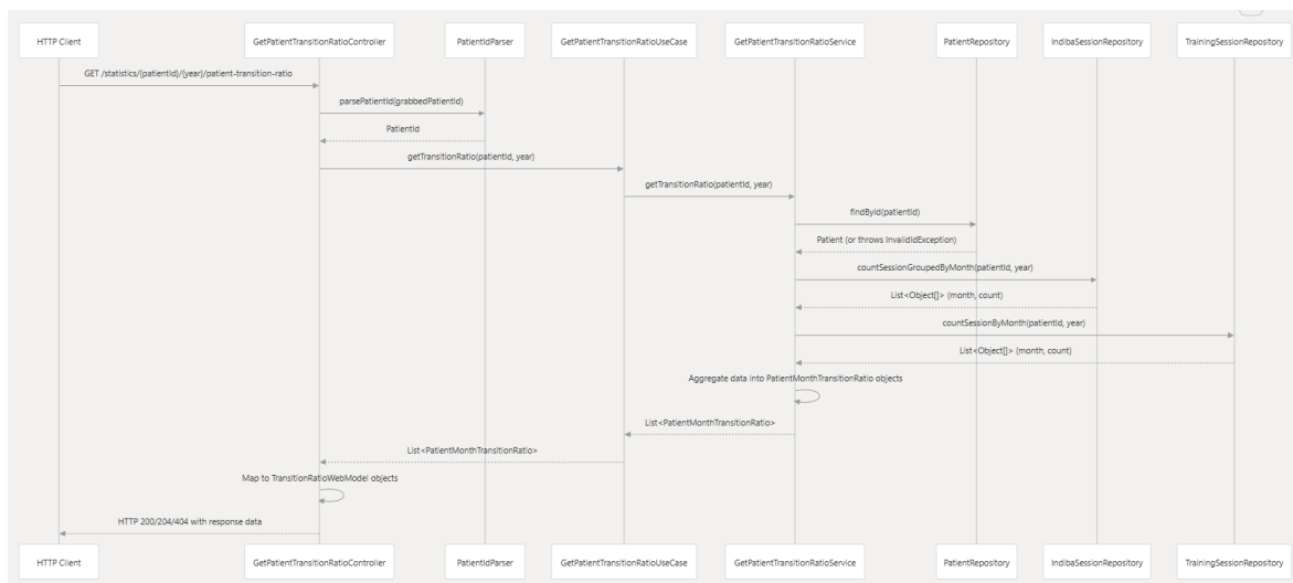
7.3.26. Flux de treball GetPatientTransitionRatio . Font: Elaboració pròpia
