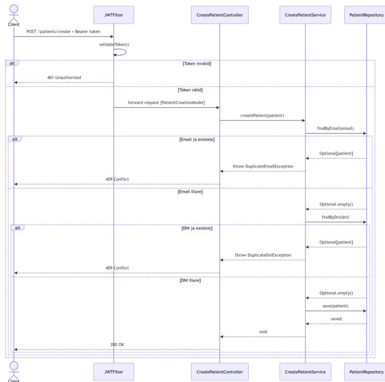
7.3.21. Flux de treball per CreatePatient. Font: Elaboració pròpia
