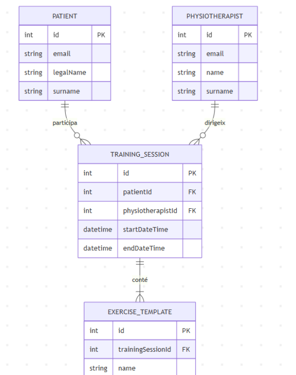
7.2.20 Diagrama d'entitat TrainingSession. Font: Elaboració pròpia
