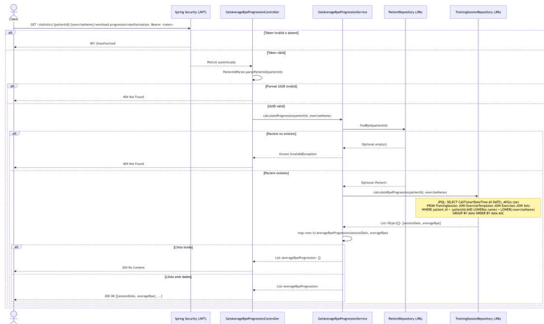
7.3.27. Diagrama de seqüència GetAverageRpeProgression . Font: Elaboració pròpia
