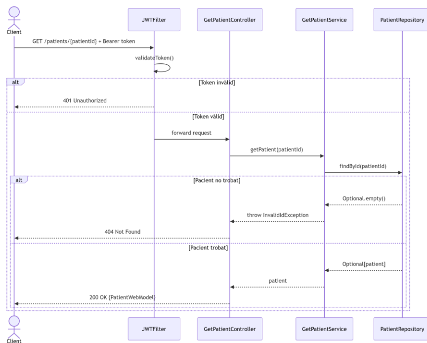
7.3.22. Flux de treball de GetPatient. Font: Elaboració pròpia
