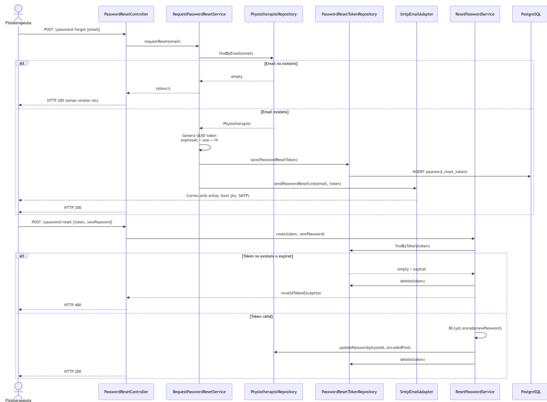
7.6.30. Flux de treball PasswordReset. Font: Elaboració pròpia
