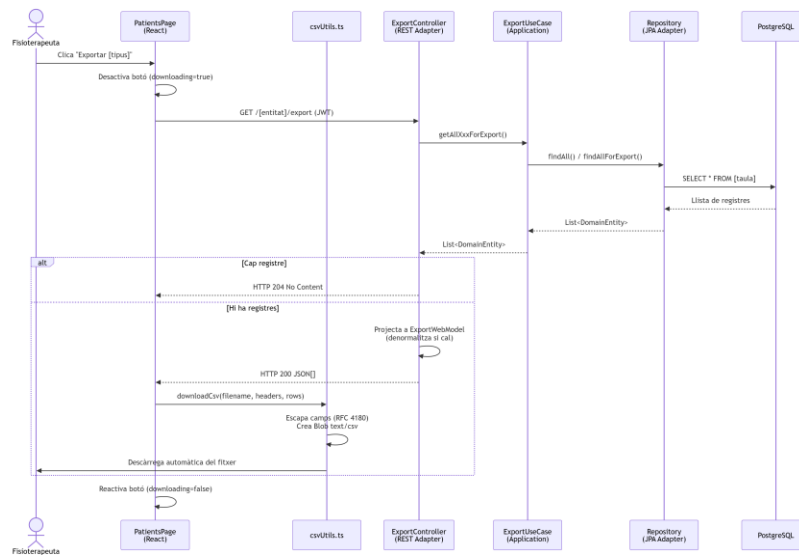
7.3.28. Flux de treball Exportació de dades a CSV. Font: Elaboració pròpia
