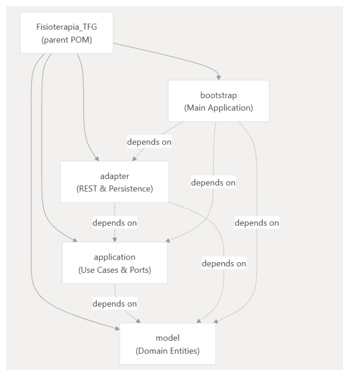
7.1.13. Diagrama Arquitectura Hexagonal del projecte. Font: Elaboració pròpia
