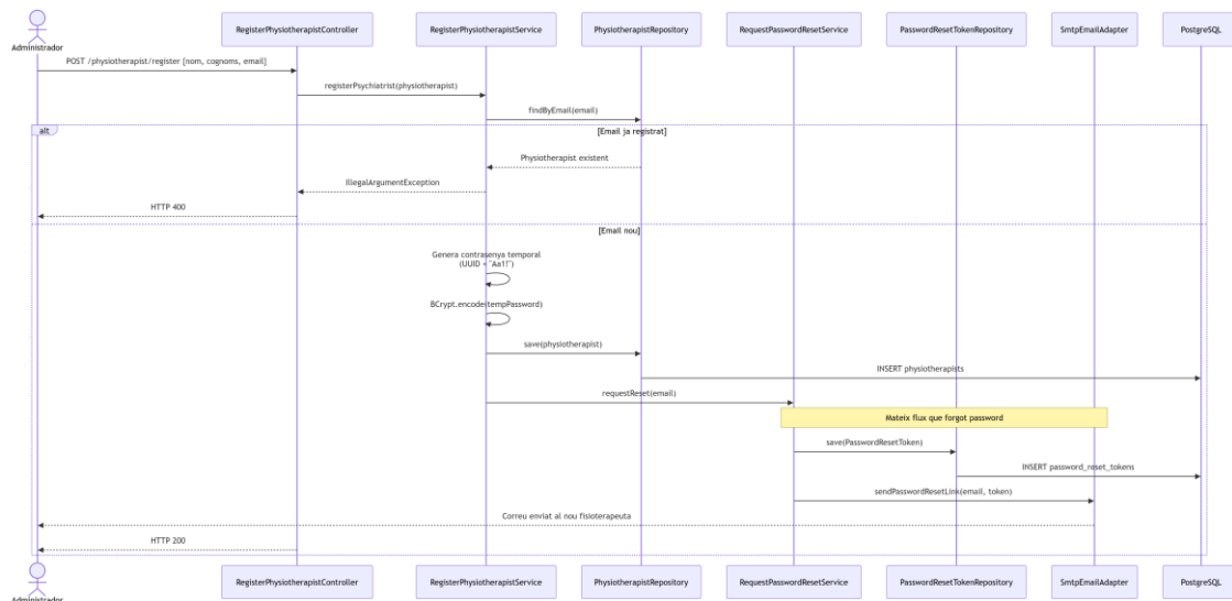
7.6.31. Flux de treball Activació de compte. Font: Elaboració pròpia
