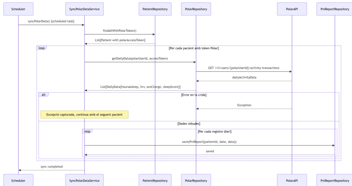
7.3.25. Diagrama de Seqüència PolarDailyScheduler. Font: Elaboració pròpia
