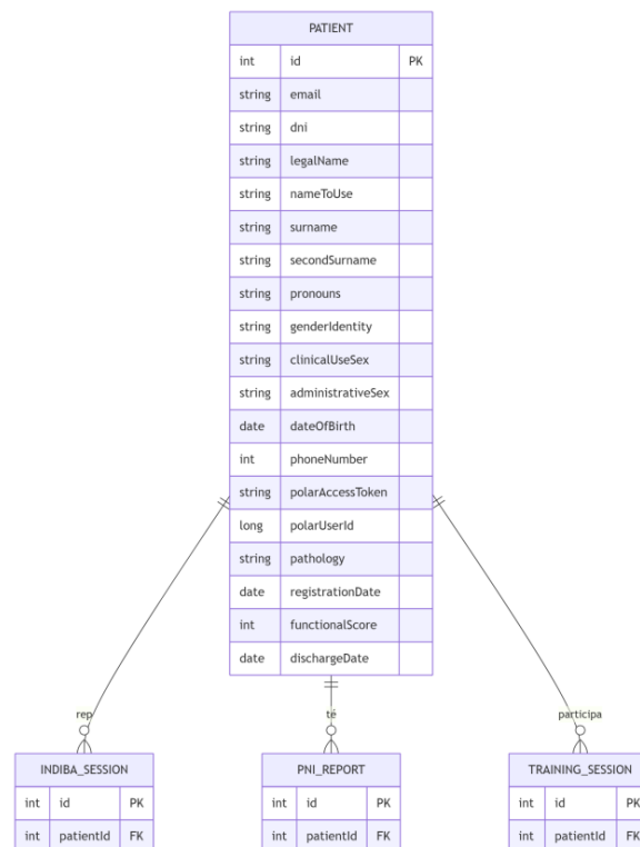
7.2.17. Diagrama d'entitat Patient. Font: Elaboració pròpia
